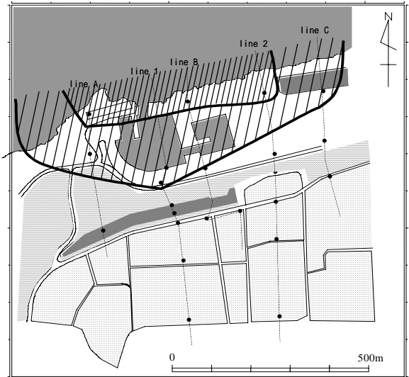
図-15 N系強風時の飛来塩分量半面分布
