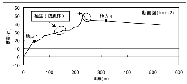
図-2 南大東漁港の断面
