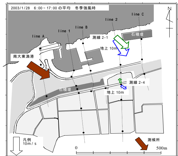
図-8 風況平面分布図 (冬季強風時)
