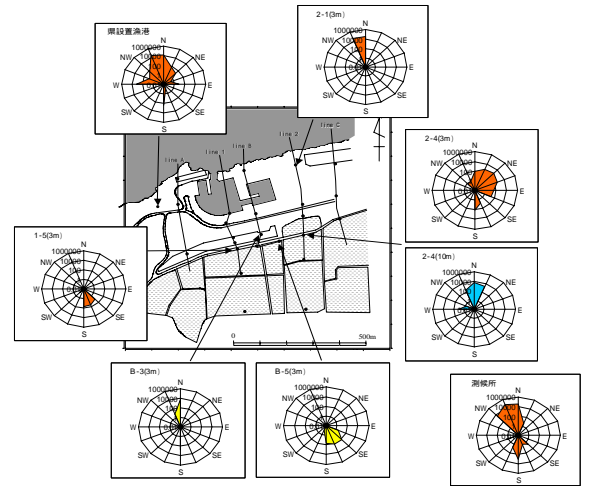
図-10 風のエネルギー分布(line-2-1: N)
