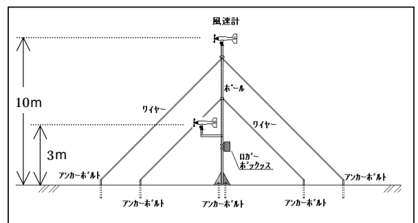
図-4 風向・風速計設置状況図
