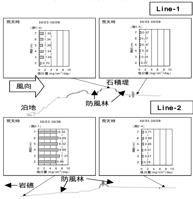
図-14 N系強風時の飛来塩分量の鉛直分布
