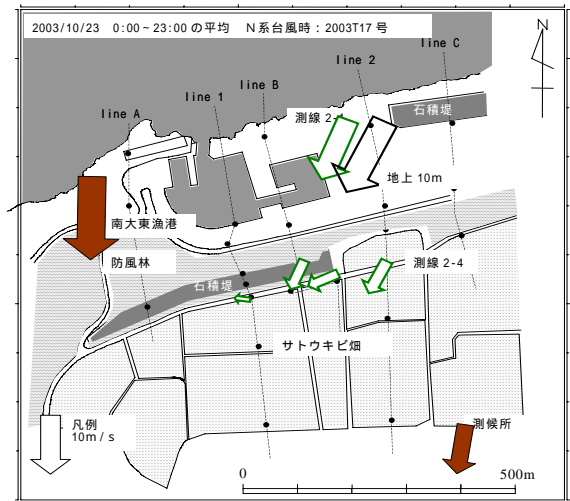
図-9 風況平面分布図（N系台風時）
