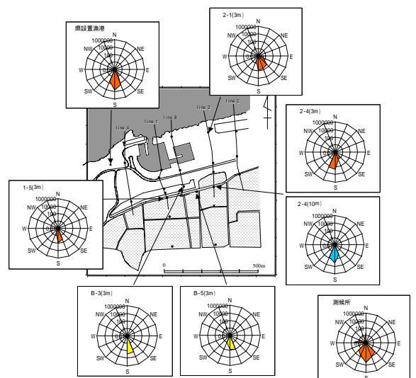
図-12 風のエネルギー分布(line-2の地点1: S)
