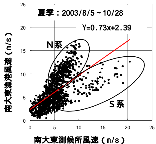
図-5 南大東漁港と南大東測候所の風速相関図
