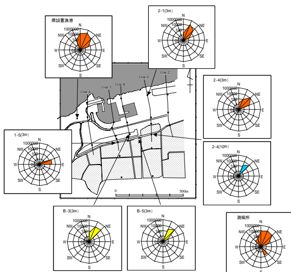
図-11 風のエネルギー分布(line-2の地点1: NE)
