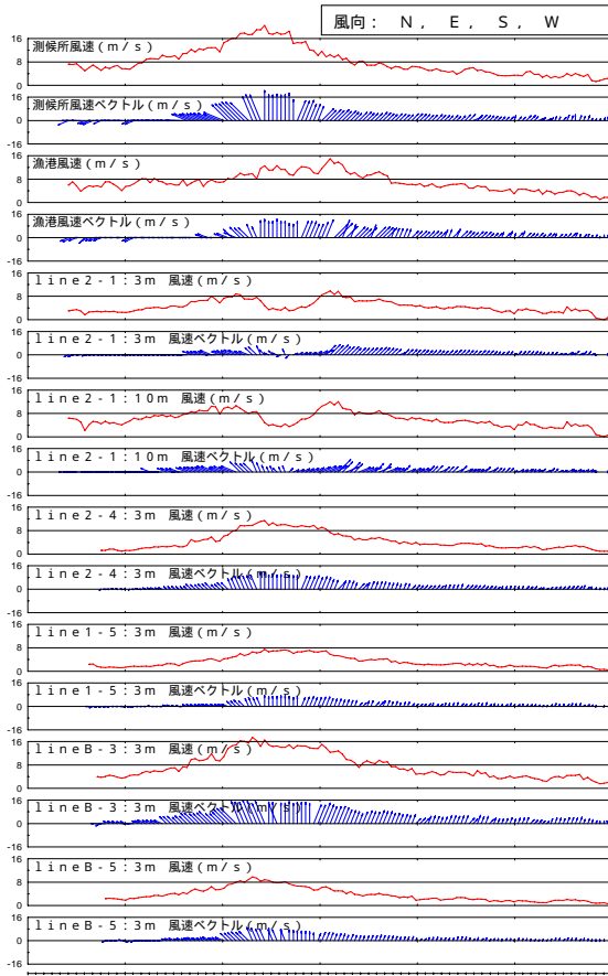
図-6 S系台風時の風況経時変化
