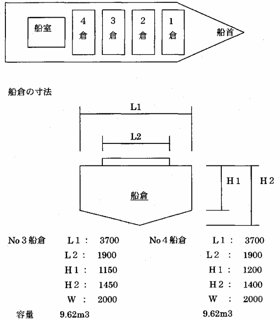
図-1 E漁船の船倉および船倉寸法
